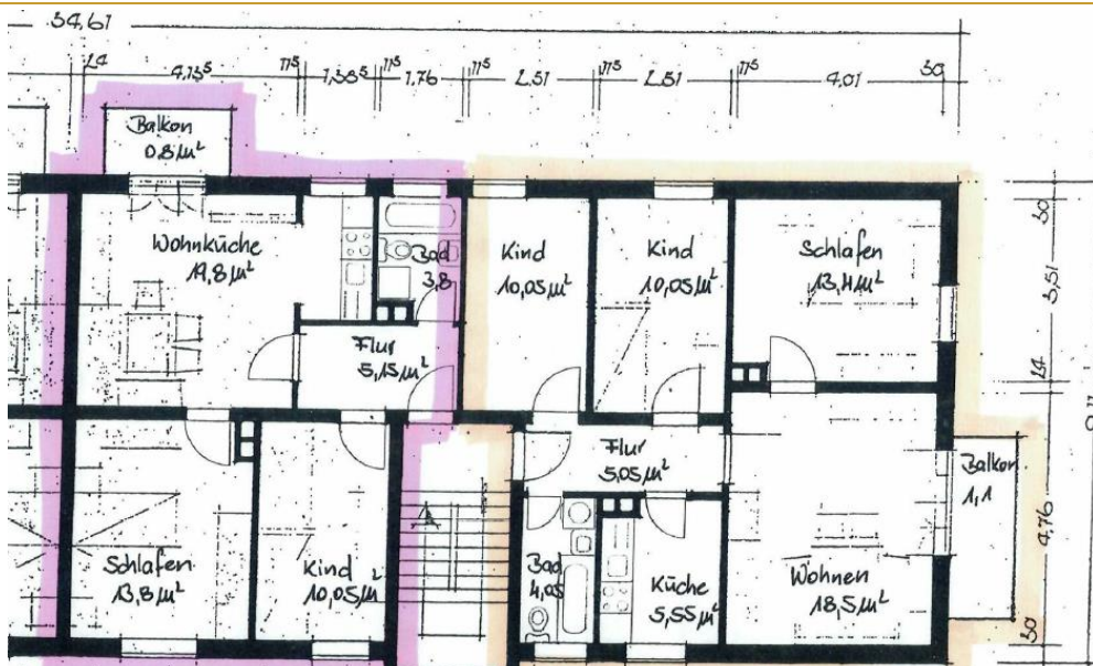
Grundriss für 3. Obergeschoss (lila)
